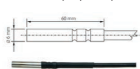
Pt1000TG68/E (-80°C až +200°C)
